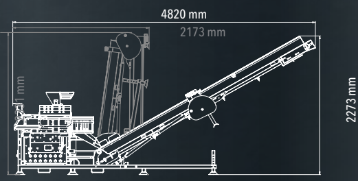
Maße Förderband 4 m
