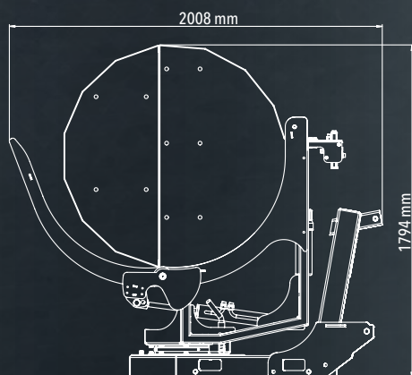
Maße 3-Punkt-Bündler eco &amp; proline, 1,0 rm
