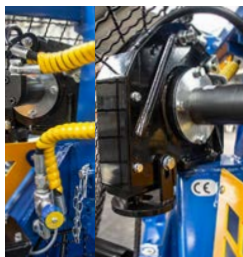
Seilausstoss inkl. Endabschalter
