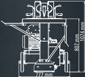
Abbildungen H8 mit Stützrad
